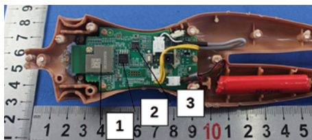
Rys. 11 Hello Barbie po rozebraniu.
